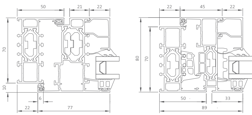
Naar buiten draaiend raam
